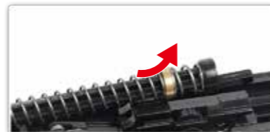
Avec précaution faites pivoter le guide de ressort et retirez-le lentement.
